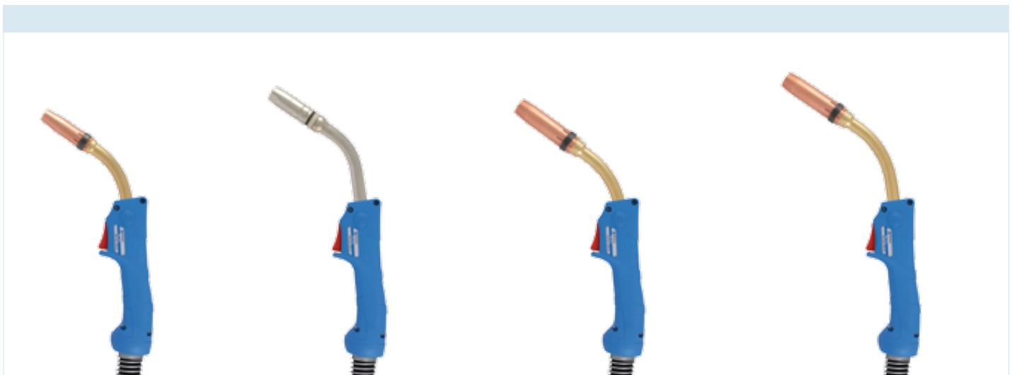
TBi 241 100% (10 min.) Mix: 270 A CO 2 : 300 A Ø 0.8-1.2 mm
