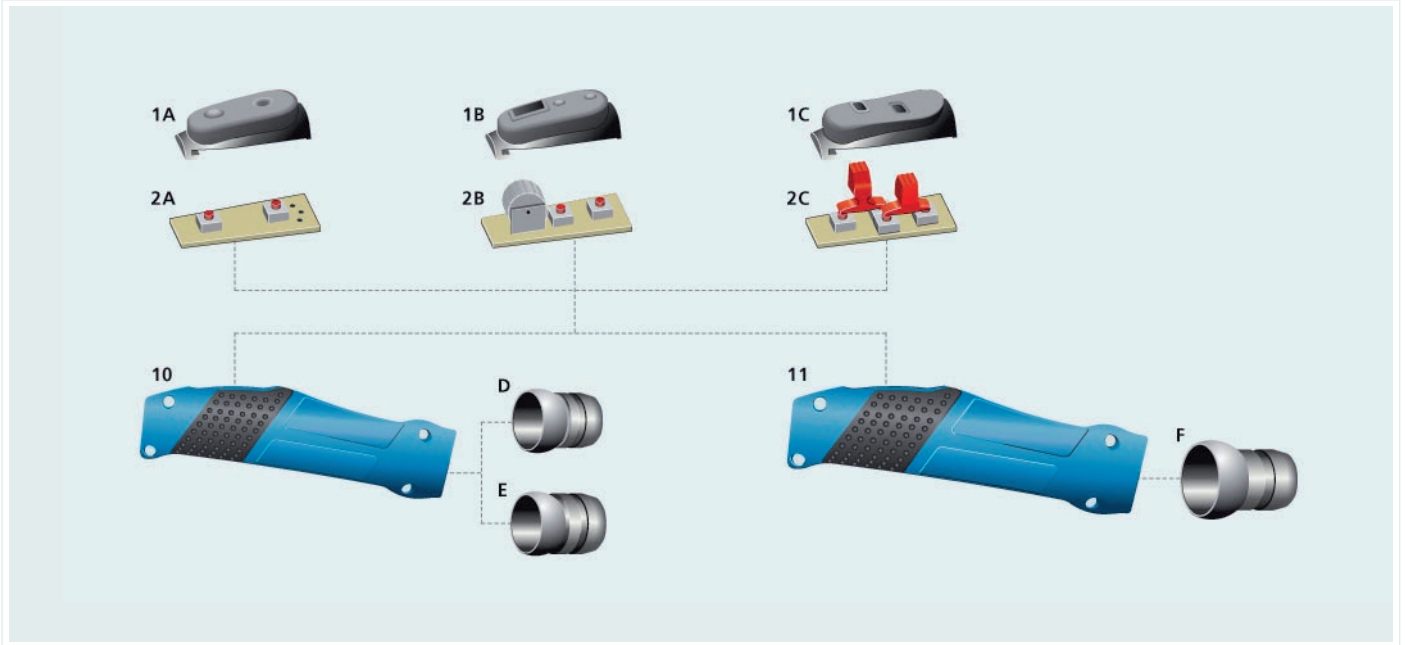
Griffe und Module / Handles and modules / Poignées et modules
