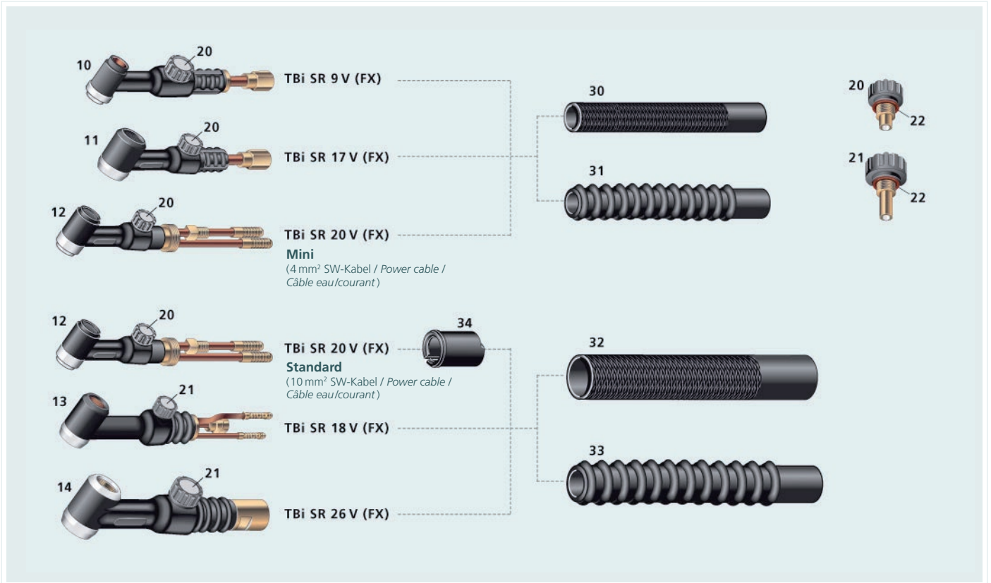
Griffrohre für Ventiltrenner / Handle tubes for torch bodies with valve / Poignées pour version à valve
