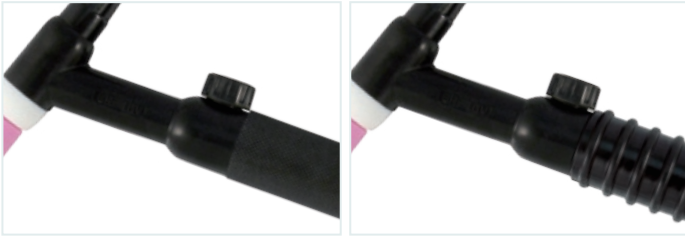
Griffrohre für Ventiltrenner / Handle tubes for torch bodies with valve / Poignées pour version à valve
